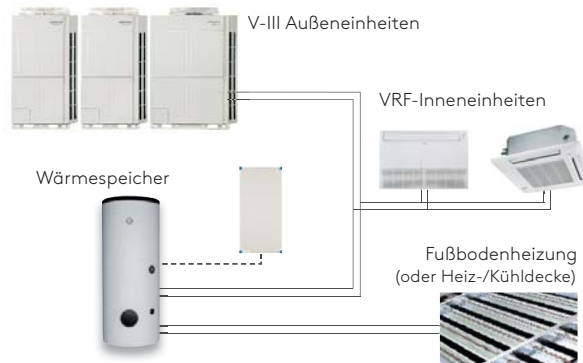
VRF-Wasserkonditionierung
