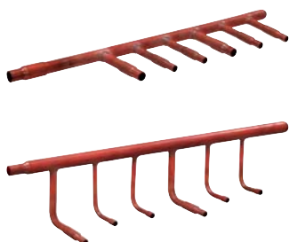
Kopfverteiler-Set 6-armig, 2-Leiter: Saugleitung (oben) Flüssigkeitsleitung (unten)
