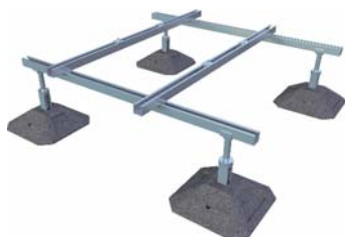
Flex-O-Frame XL Höhenverstellbares Aufstellsystem mit Schwingungsdämpfung
